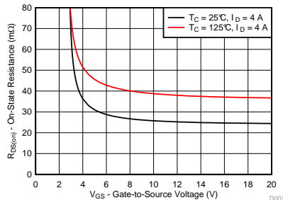
R_{DS(on)} 与 V_{GS} 间的关系
